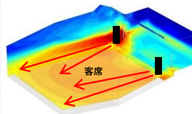
合成音圧レベル分布図
